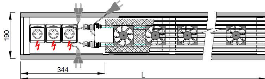
FBO-QE-215E-175-L-190
