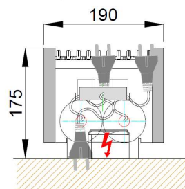
FBO-QE-215E-175-L-190
