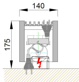
FBO-QE-115E-175-L-140
