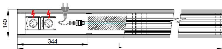
FBO-QE-115E-175-L-140
