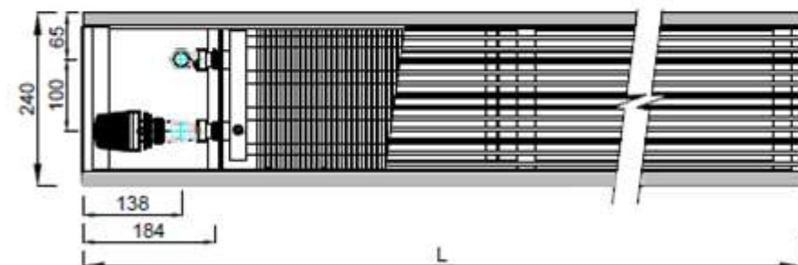
FBO-1020-175-L-240
