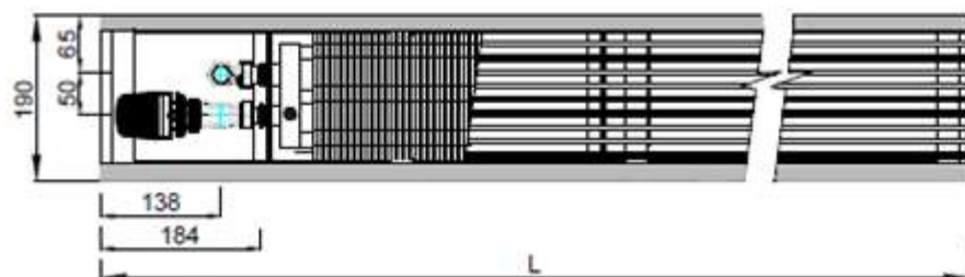
FBO-1015-175-L-190
