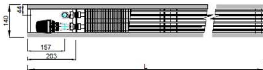
FBO-1010-175-L-140
